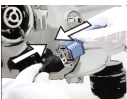
4- CONECTE RESPEITANDO AS POLARIDADES, RECONECTE OS PARAFUSOS E A VEDAÇÃO.
